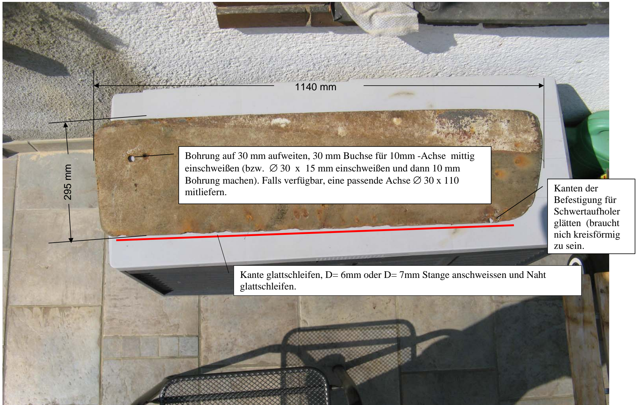
Erforderliche Reparaturarbeiten Schwert, Flying Cruiser S - „Anansi“ . Das Schwert ist aus 7 mm Stahl, verzinkt und an den Kanten und Bohrungen korrodiert.
